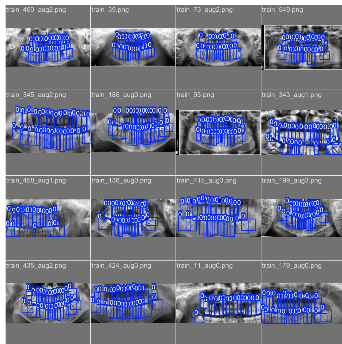
train_batch1.jpg
