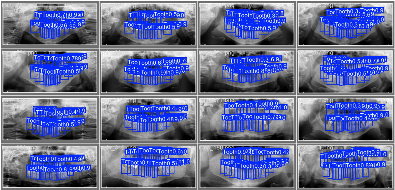
val_batch0_pred.jpg
