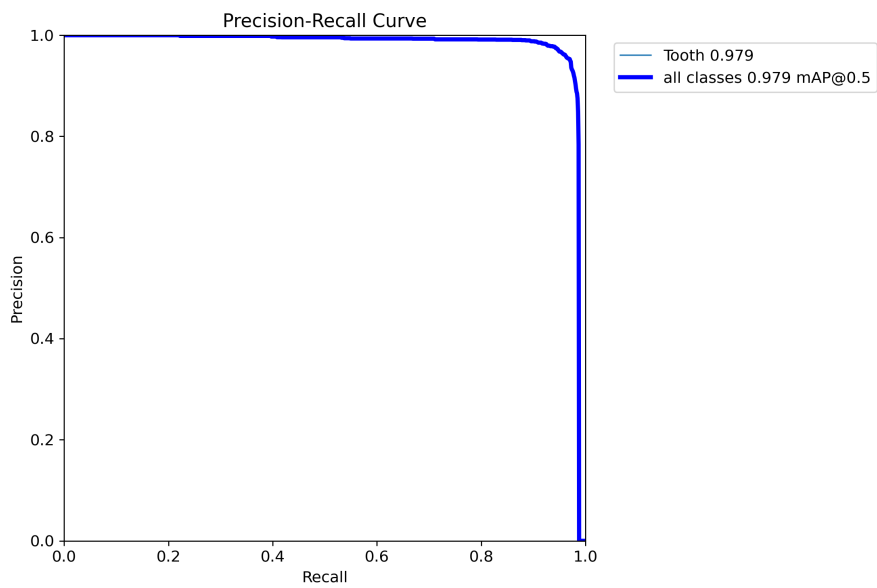
BoxPR_curve.png
