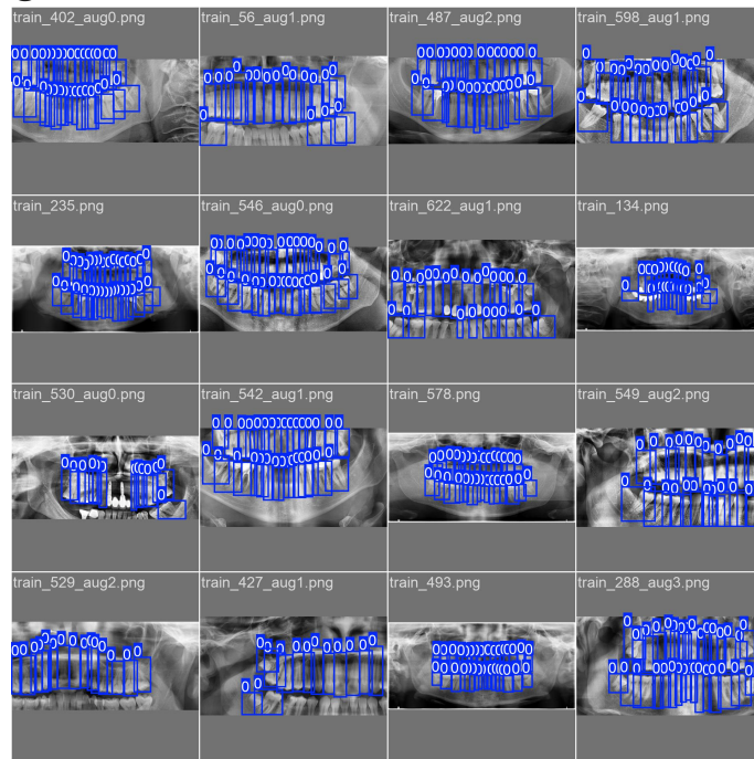
train_batch0.jpg
